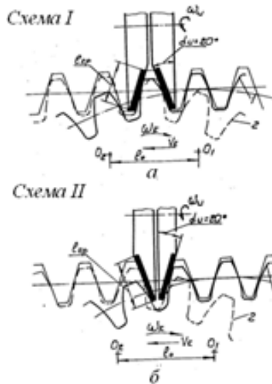
Рис. 7 – Технологические схемы резания дисковыми немодульными фрезами: a – схема одновременной обработки двух профилей одного зуба, б – схема одновременной обработки двух профилей соседних зубьев
