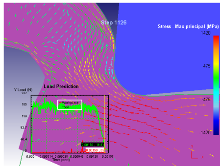
Рис. 3 – Распределение интенсивности напряжений в области формообразования поверхностного слоя
